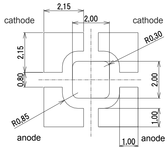
■推奨取り付けパターン
