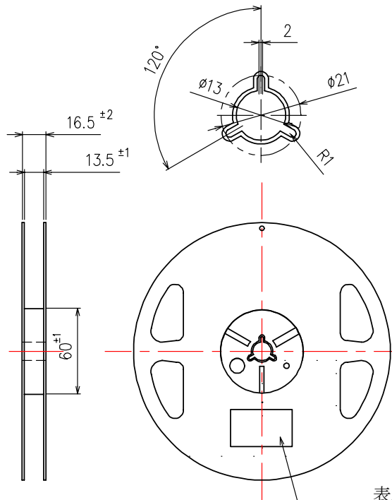
リールセンター穴拡大図
