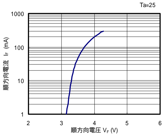
順方向電圧 - 順方向電流特性
