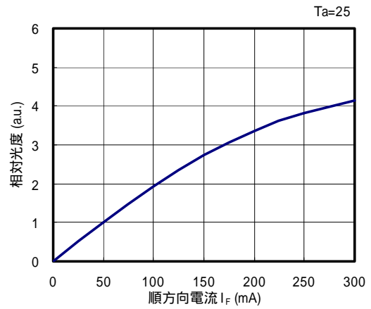
順方向電流 - 相对光度特性
