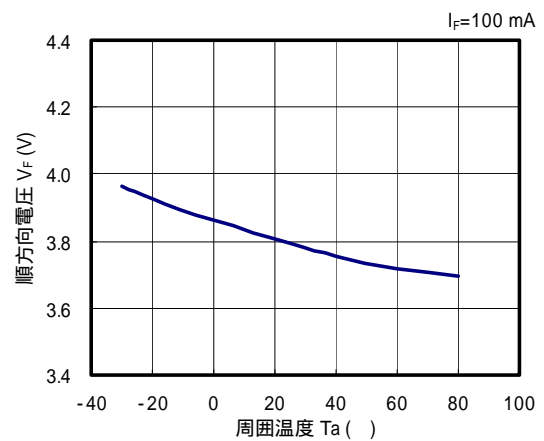
周囲温度 - 順方向電圧特性
