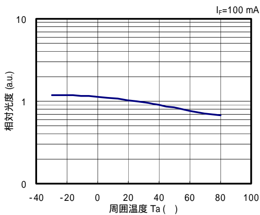
周囲温度 - 相对光度特性
