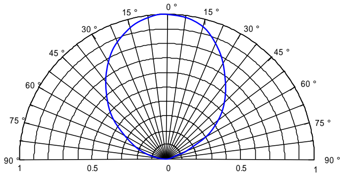
指向特性
